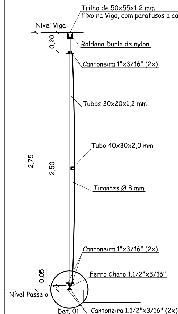
Corte A-A
