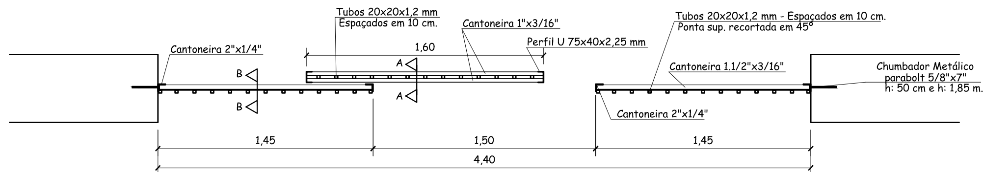
Planta Baixa
