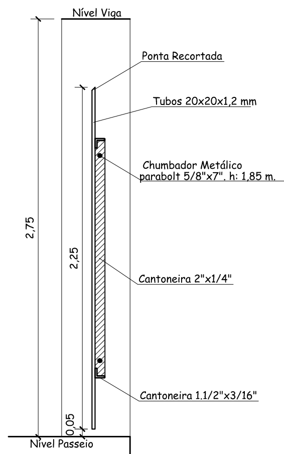
Corte B-B
